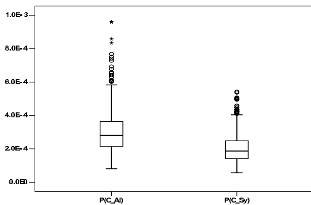
شکل ۱۸. ASE برآوردگرهای مرکب با w_i^*
